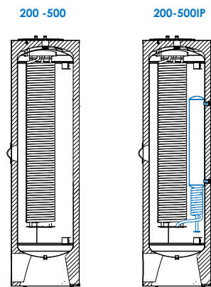
ACS + INERCIA ACS + INERCIA + 1 SERPENTÍN
