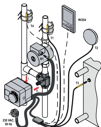
Montaje en válvula
