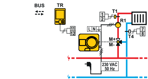
Esquema 360b Circuito de calefacción adicional
