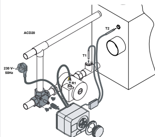
Montaje en válvula
